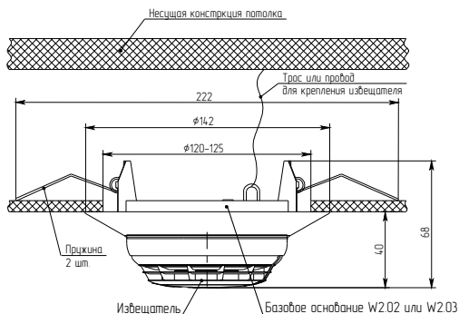
Рисунок 2 – Установка извещателя на подвесном потолке
