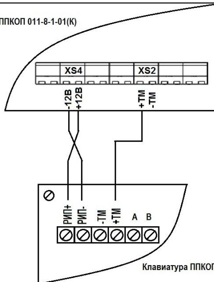
Рисунок 5. Схема подключения клавиатуры к приборам ППКОП 011-8-1-01К, -02К, -041К, -061К, -064-1К, -01К-ТСР
