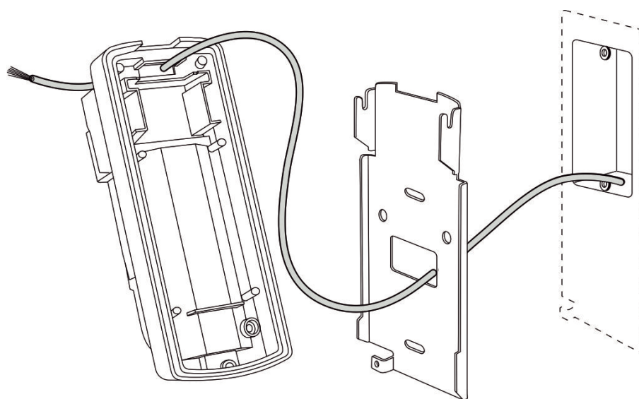
Рисунок 2.9 - Прокладка кабеля
