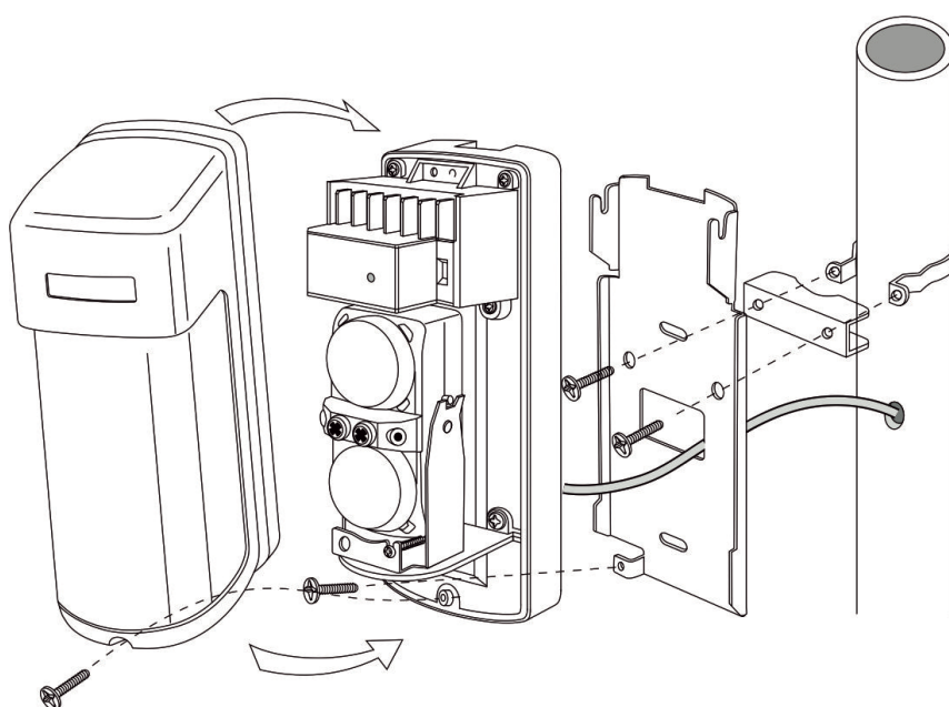
Рисунок 2.12 - Последовательность установки кронштейна на монтажную трубу
