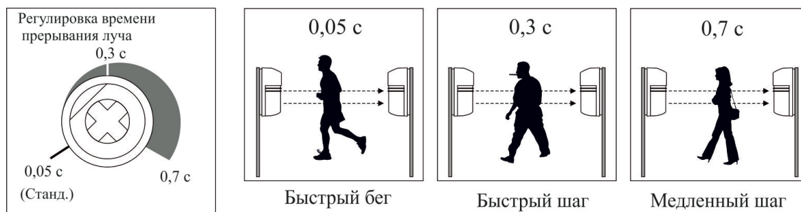
Рисунок 2.20 - Выбор времени прерывания луча
