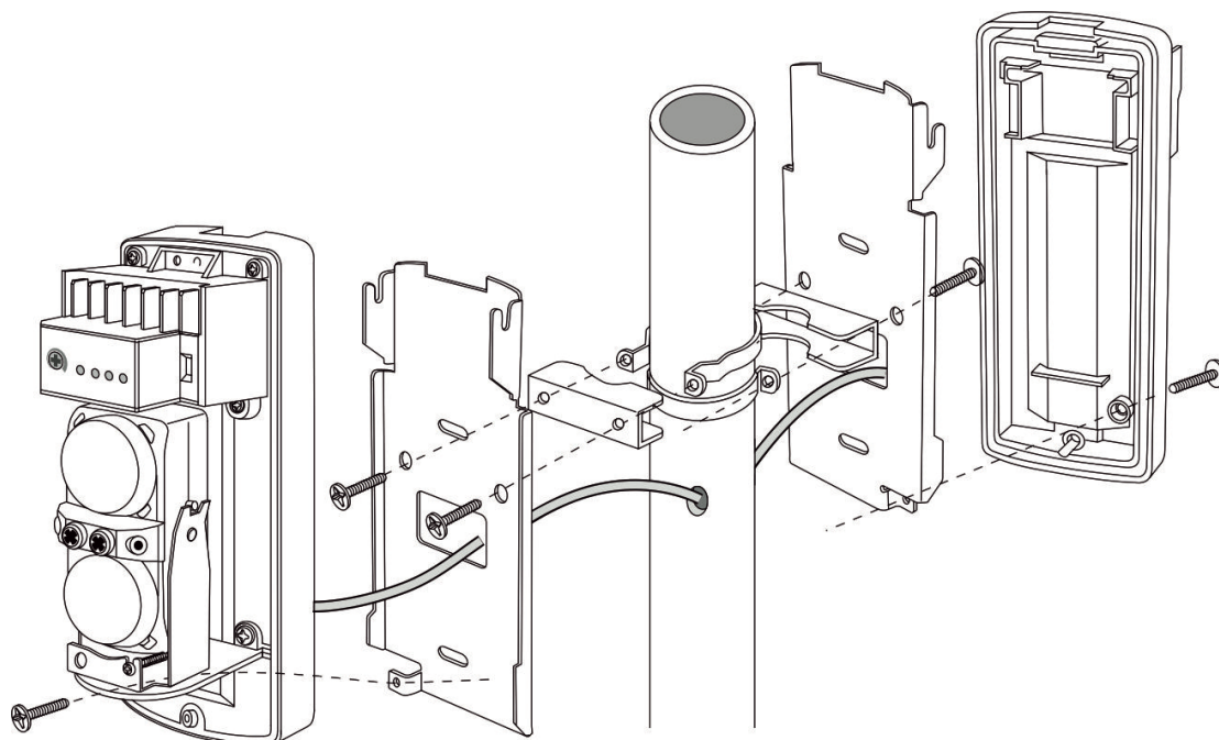
Рисунок 2.13 - Одновременная установка на монтажную трубу двух изделий
