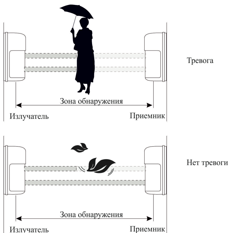
Рисунок 1.3 - Принцип действия извещателя
