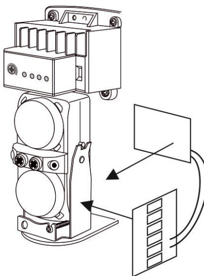
Рисунок 1.7 - Крепление плат модуля подогрева
