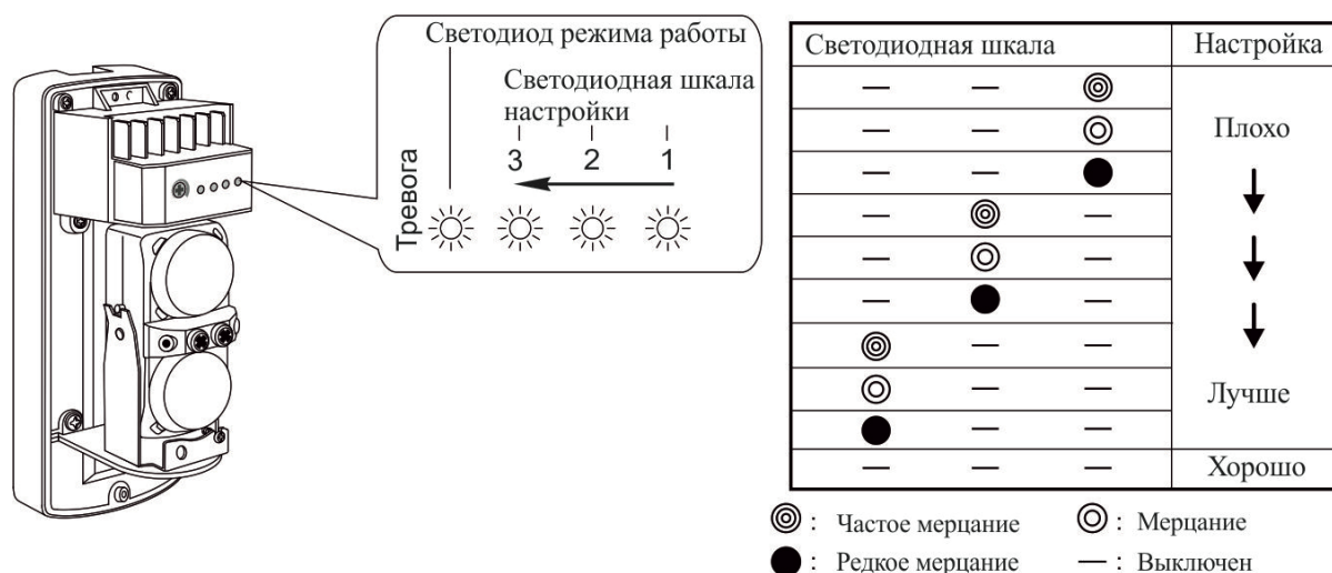
Рисунок 2.18 - Светодиодная шкала настройки
