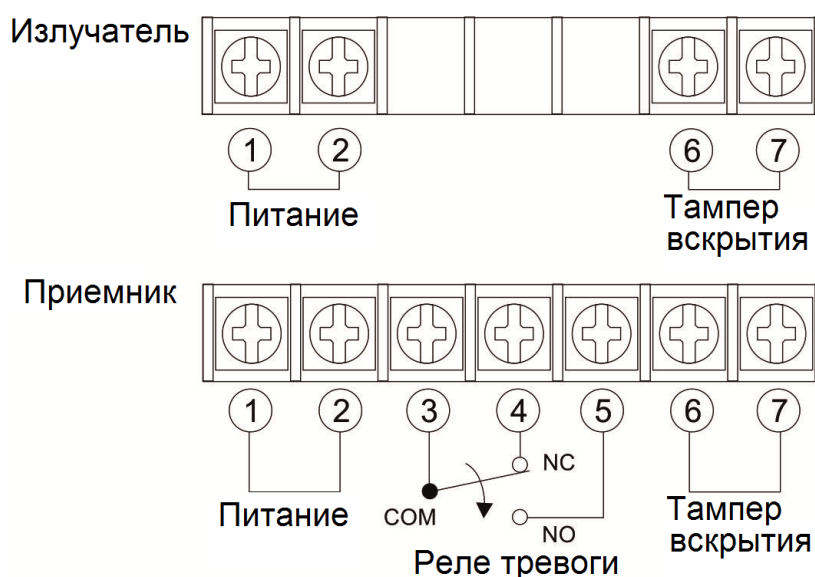
Рисунок 1.1 - Расположение контактов на клеммных колодках приемника и излучателя
