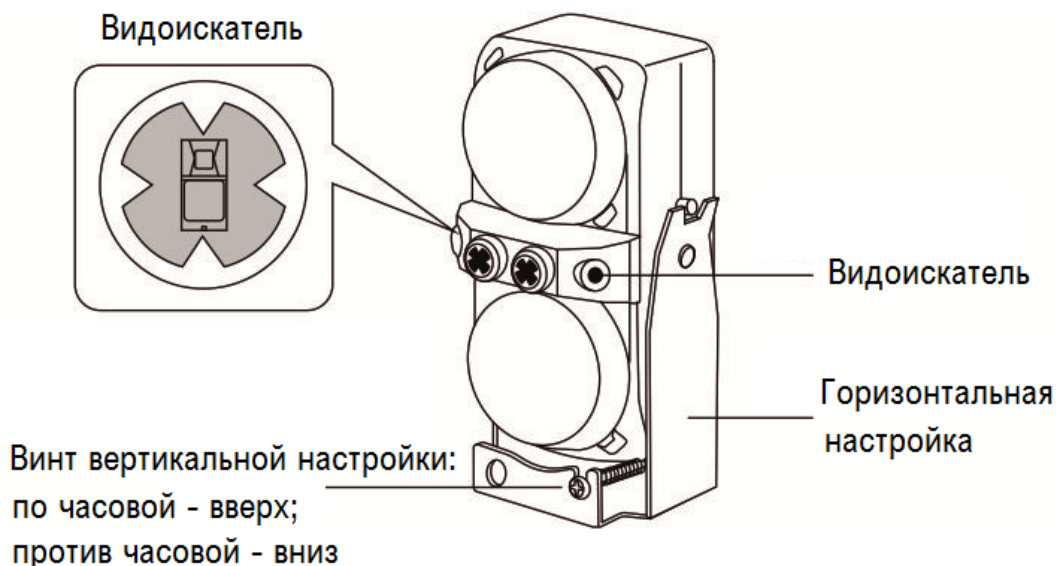
Рисунок 2.17 - Оптический узел
