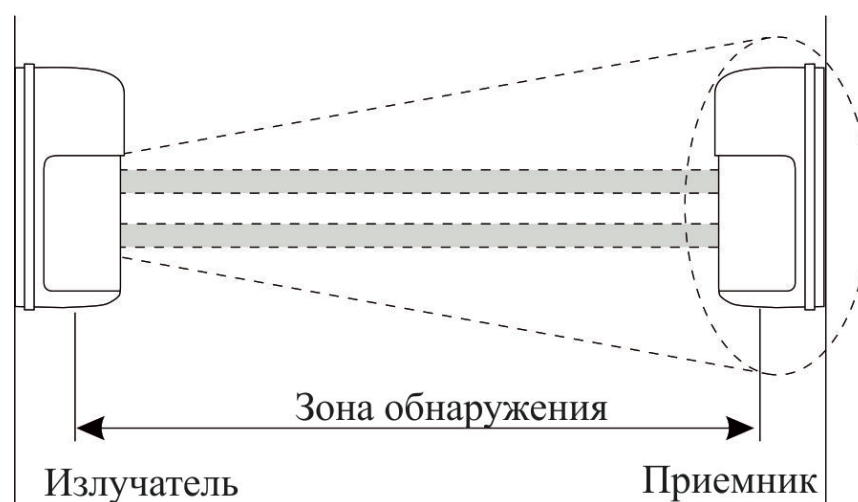
Рисунок 1.2 - Расположение БИ и БП при формировании ИК барьера
