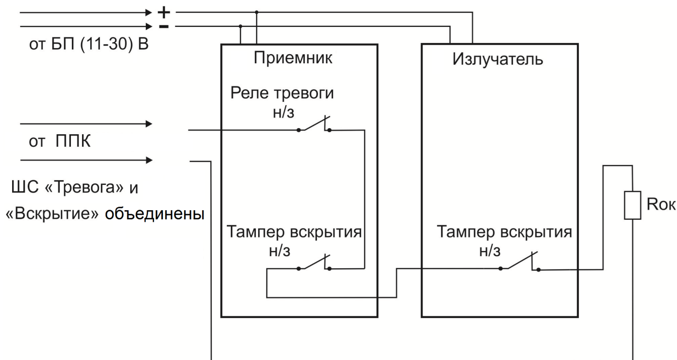
Рисунок 2.15 - Схема соединения извещателя с ППК по четырехпроводному шлейфу
