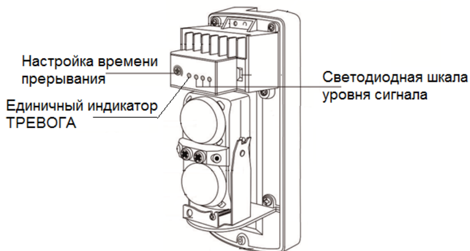
Рисунок 2.19 - Положение органов регулировки и настройки приемника
