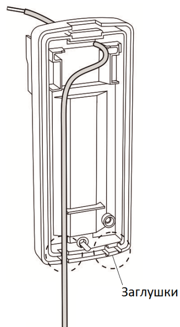
б) проводка через нижнюю часть корпуса
