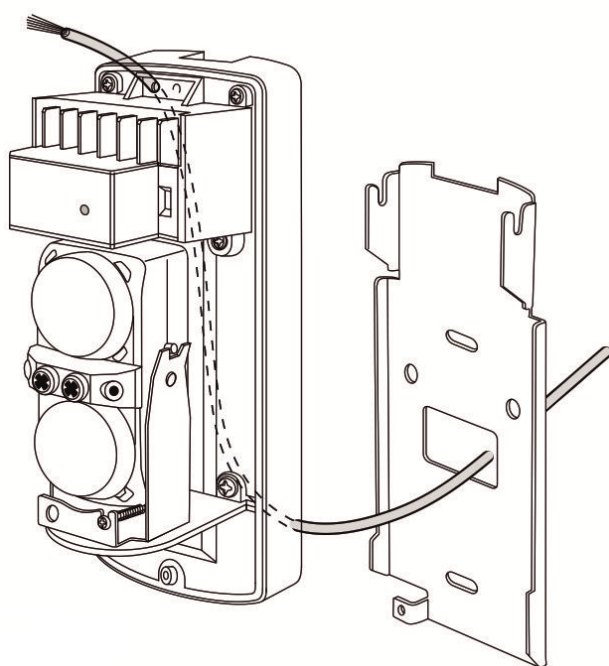
а) проводка через кронштейн
