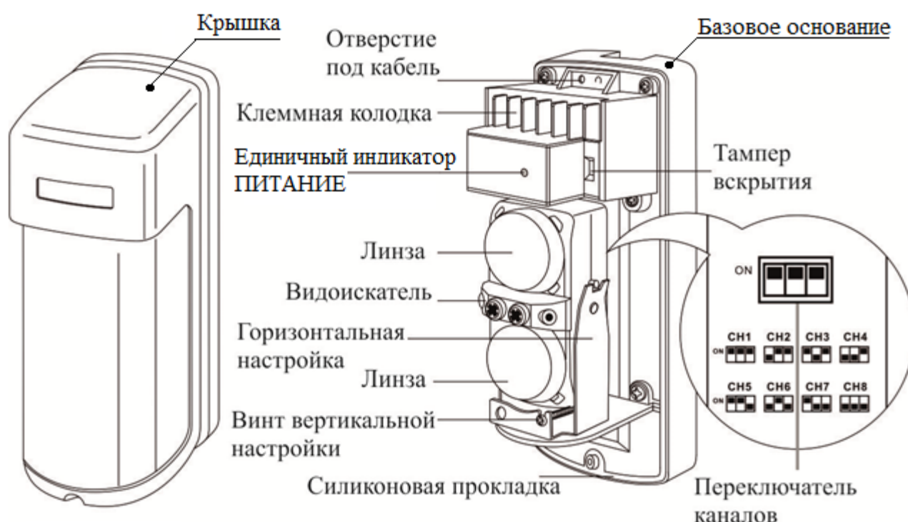
Рисунок 1.4 - Общий вид излучателя
