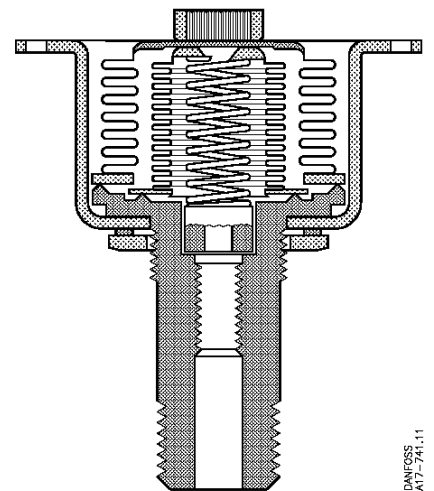
Рис.8а. Чувствительный элемент RT32W.
