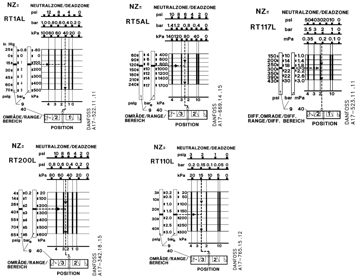
Рис.11. Диаграммы настройки
