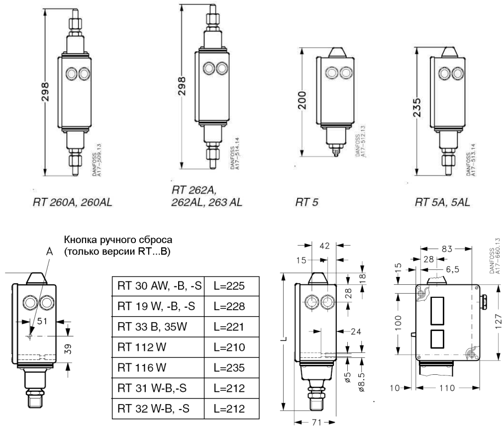
Рис.16. Габаритные размеры
