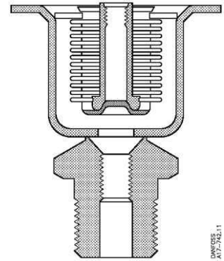
Рис.8а. Чувствительный элемент RT32W.
