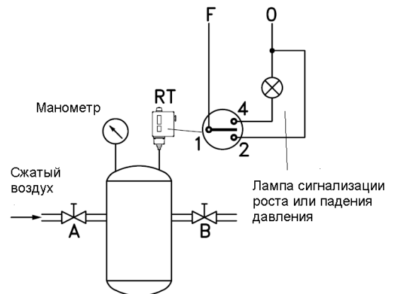
Рис.12. Пример использования реле давления с нейтральной зоной
