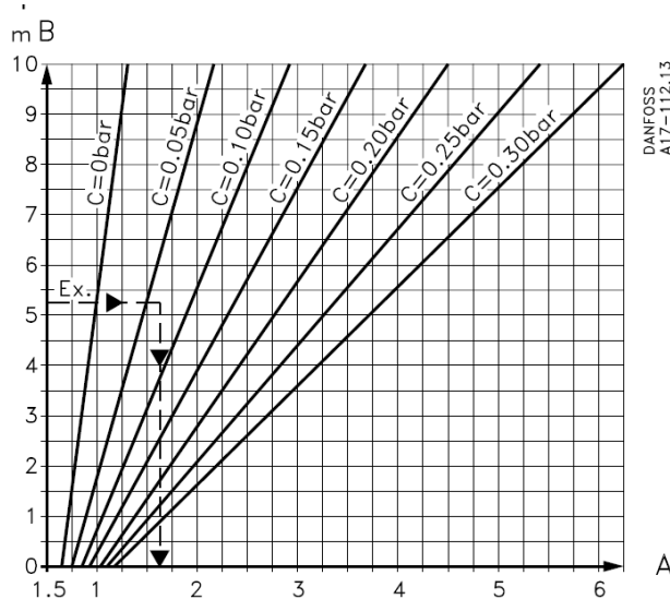
Рис.7. Диаграмма зависимости горизонтального участка A трубы от вертикального участка B
