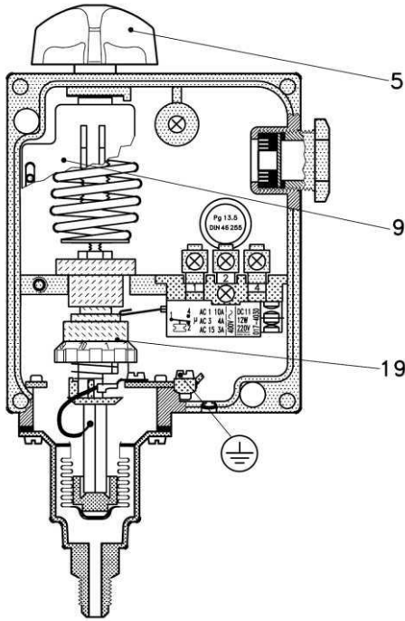
Рис.4. Настройка реле давления
