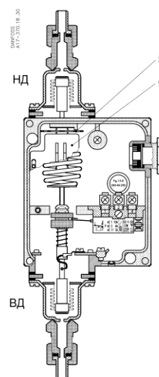
Рис. 14. Настройка реле давления
