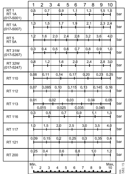
Рис.5. Диаграмма выбора дифференциала
