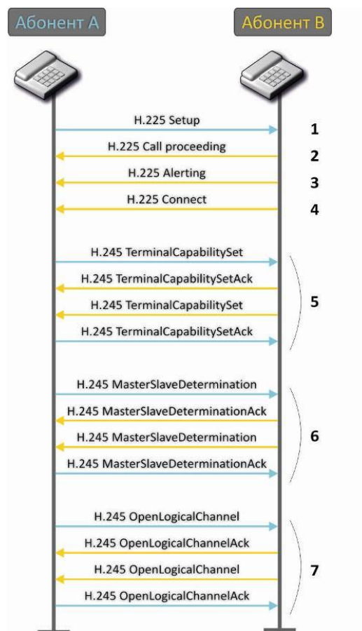
Рисунок 19 – Алгоритм вызова по протоколу H.323
