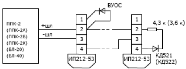
Рисунок 6 - Схема подключения извещателя ИП212-53 к пультам типа ППК-2
