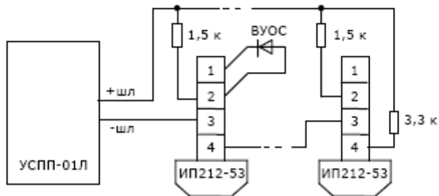
Рисунок 8 - Схема подключения извещателя ИП212-53 к прибору УСПП-01Л «Сигнал-42-01»
