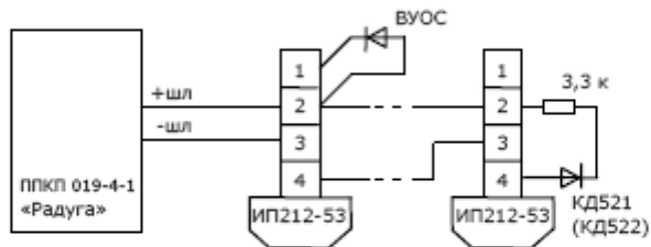
Рисунок 7 - Схема подключения извещателя ИП212-53 к прибору ППКП 019-4-1 «Радуга»
