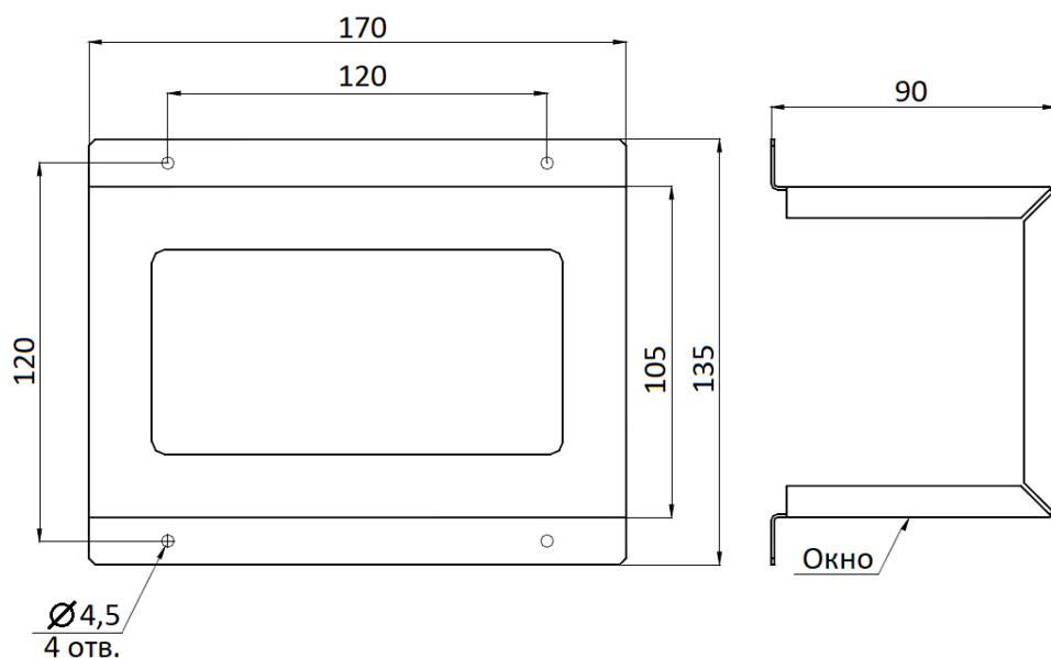
Рисунок 2 - Габаритные размеры защитного кожуха
