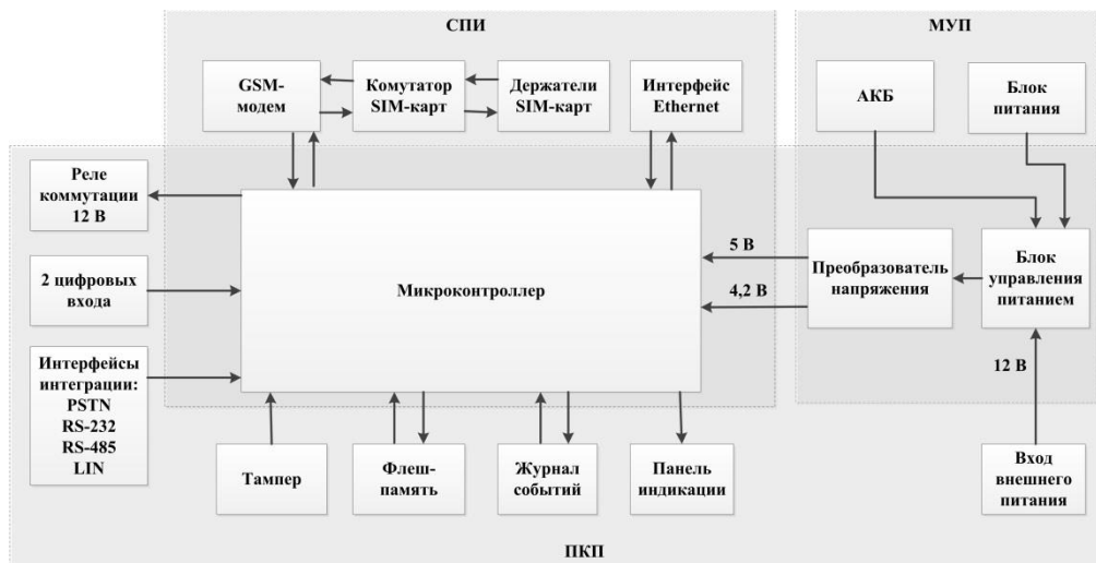
Рис. 3.1. Функциональная схема 3
