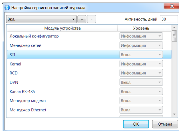
Рис. 6.9. Окно Настройка сервисных записей журнала
